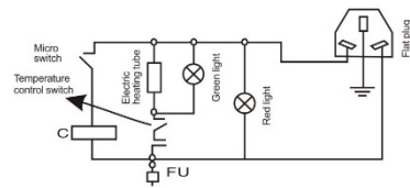
1 фаза 220В
