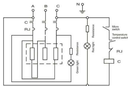
3 фазы 380В
